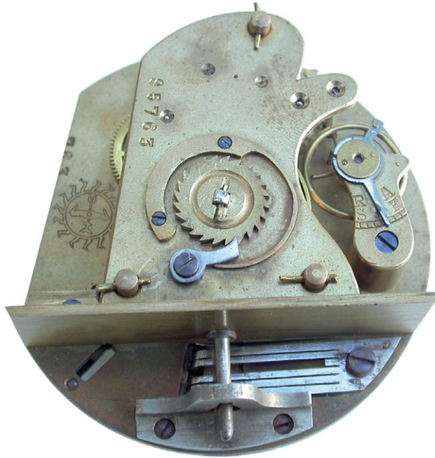
Abb. 2: Uhrwerk Typ 1. Eine der Federspitzen ist abgebrochen. Das links erkennbare Warenzeichen ließ sich Isgus 1897 schützen.
