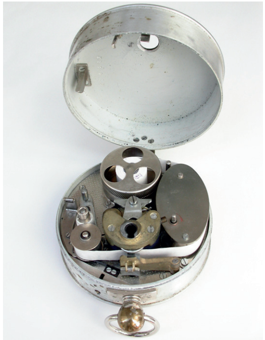
Abb. 17: Wächteruhr Typ Nr. 50.
