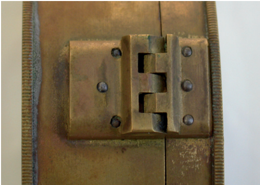
Abb. 13: Gehäusescharnier Typ 20.
