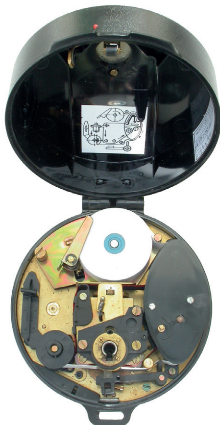
Abb. 18: Wächteruhr Typ Nr. 60.
